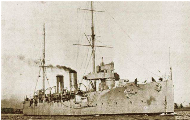
“肇和”号训练巡洋舰
