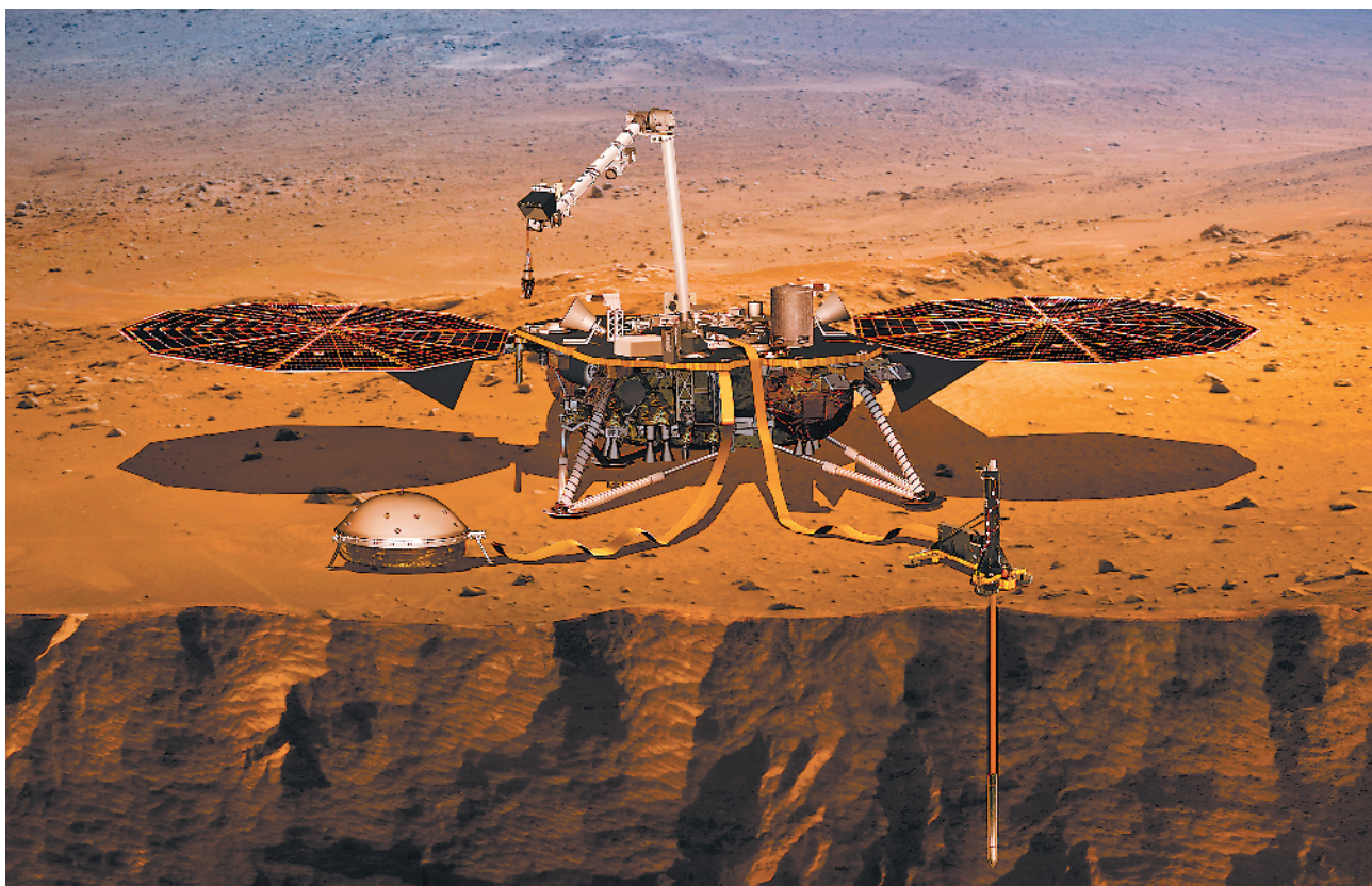
历经6个多月的航行,“洞察”号无人探测器终于抵近日地——火星。美国航天局11月21日宣布,“洞察”号计划于本月26日在火星着陆。按照计划,“洞察”号将于美国东部时间26日15时(北京时间27日4时)在火星着陆。这个有着“三条腿、一根手臂”的火星新访客抵达后,将展开两个圆形可折叠太阳能板,伸展机械臂,利用地震调查、温度测量等方法探测火星的地质构成。图为美国航天局2018年发布的“洞察”号无人探测器在火星进行钻探实验的示意图。 新华社发
