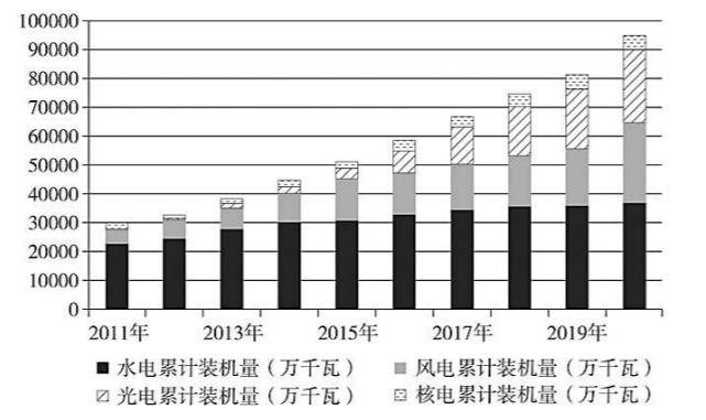
图2 2011—2020年中国非化石能源发电装机容量
