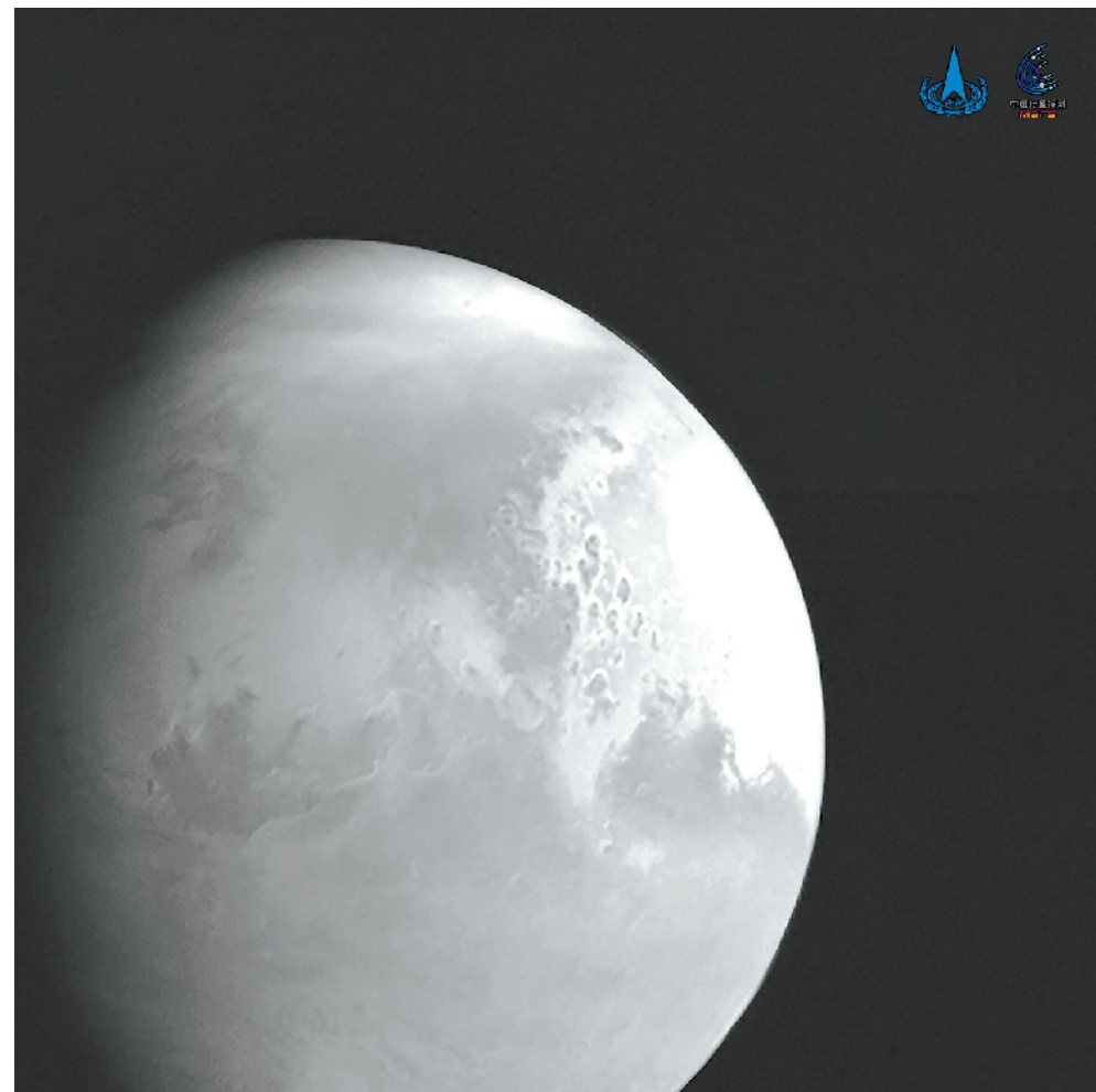
右图：国家航天局公布的“天问一号”在距离火星约220万公里处获取的首幅火星图像。
